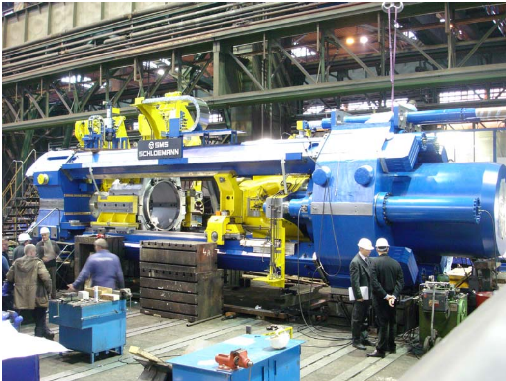
Photo : la nouvelle presse à extrusion en cours de montage
